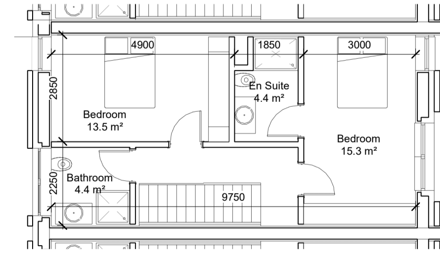
13 TH TYPE 8h (Lv02) 1 : 100
