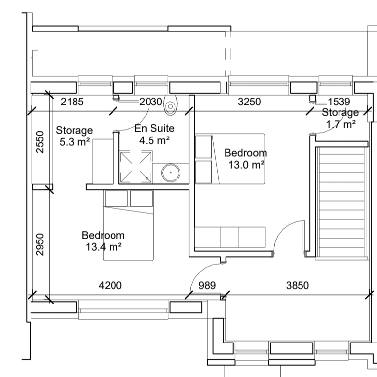
9 TH TYPE 5h (Lv02) 1 : 100
