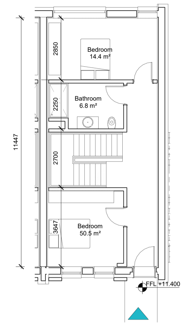
5 TH TYPE 3h (GF) 1 : 100
